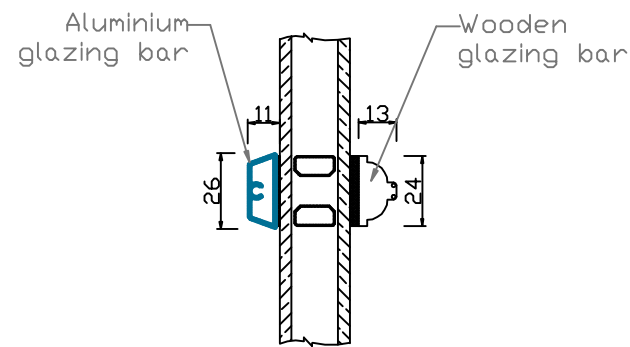
GLAZING BAR
